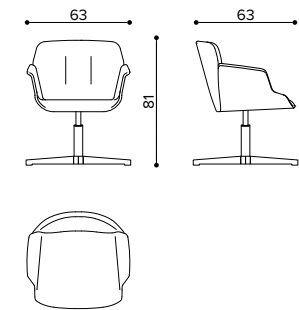
HV 6098 4 stars aluminium base - base 4 razze alluminio
